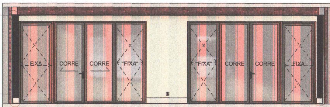
02 ELEVÇÃO 04 1 : 50
