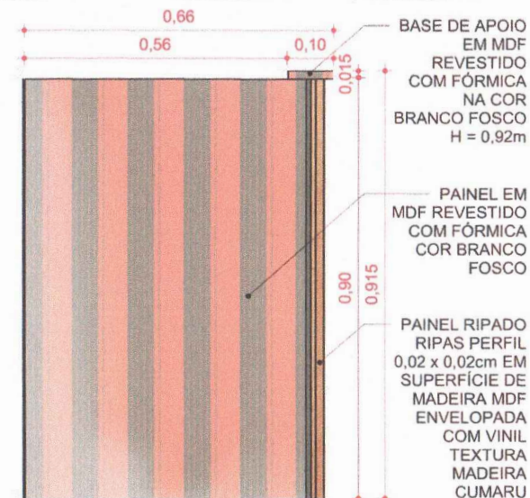
04 VISTA ESQUERDA 1 : 10
