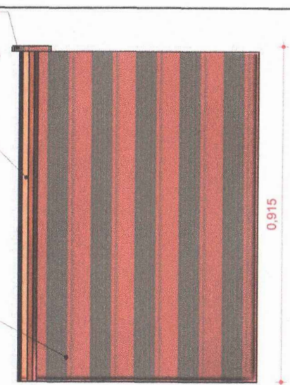
04 VISTA ESQUERDA 1 : 10
