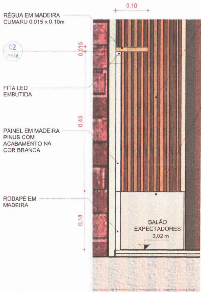
01 DETALHE - D11 1:5
