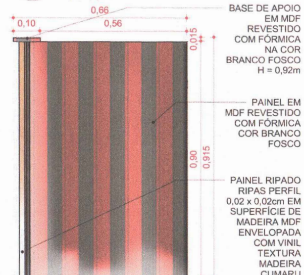
05 VISTA DIREITA 1 : 10
