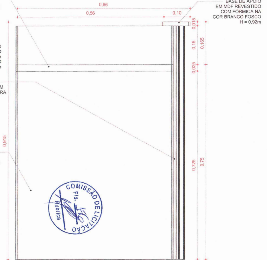
02 CORTE TRANSVERSAL 1:5
