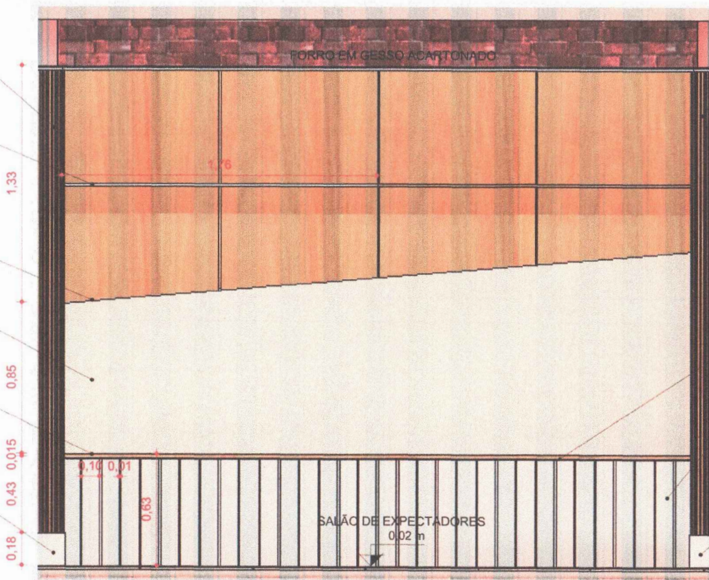
01 DETALHE - D07 1 : 20
