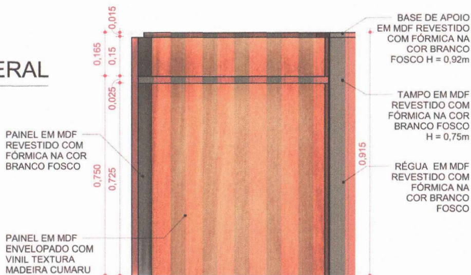
03 VISTA POSTERIOR 1 : 10
