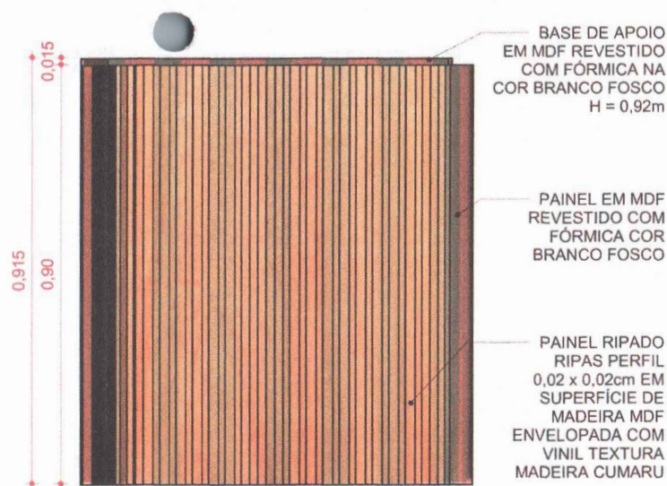
02 VISTA FRONTAL 1 : 10
