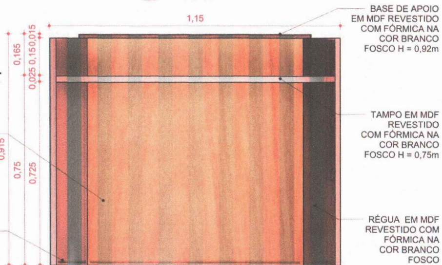
03 VISTA POSTERIOR 1 : 10
