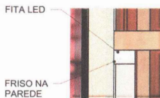
02 DETALHE - D12 1:2
