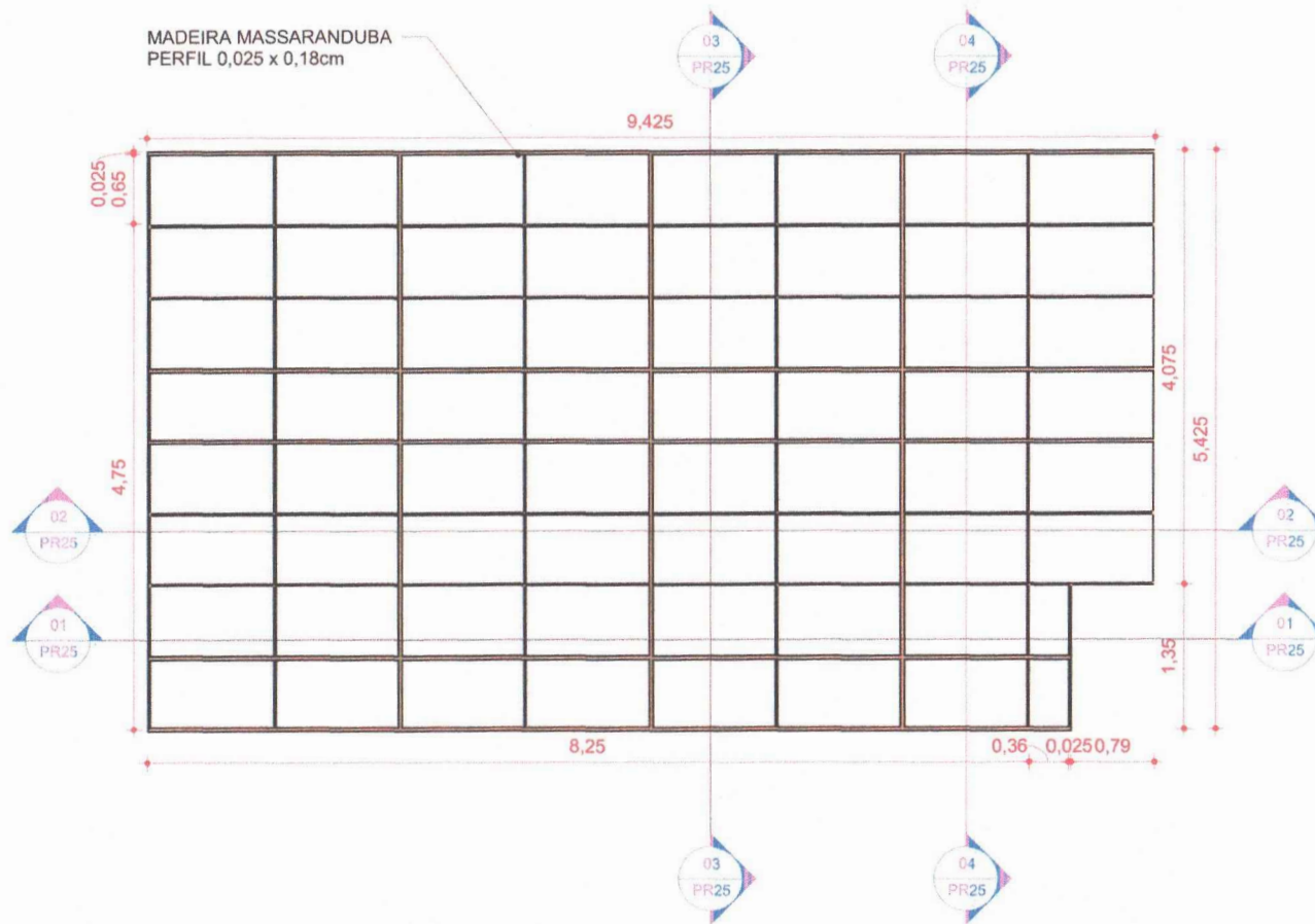
02 PLANTA DE DETALHE 1 : 50
