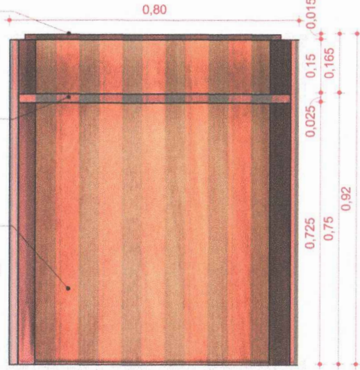
03 VISTA POSTERIOR 1 : 10
