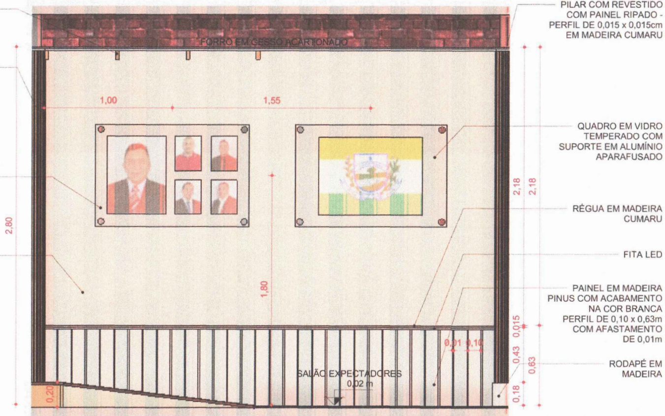
01 DETALHE - D09 1 : 20
