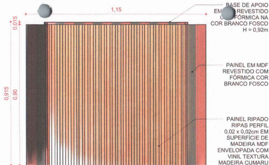
02 VISTA FRONTAL 1 : 10
