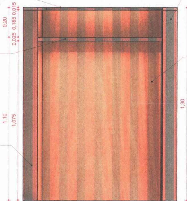
01 VISTA POSTERIOR 1 : 10
