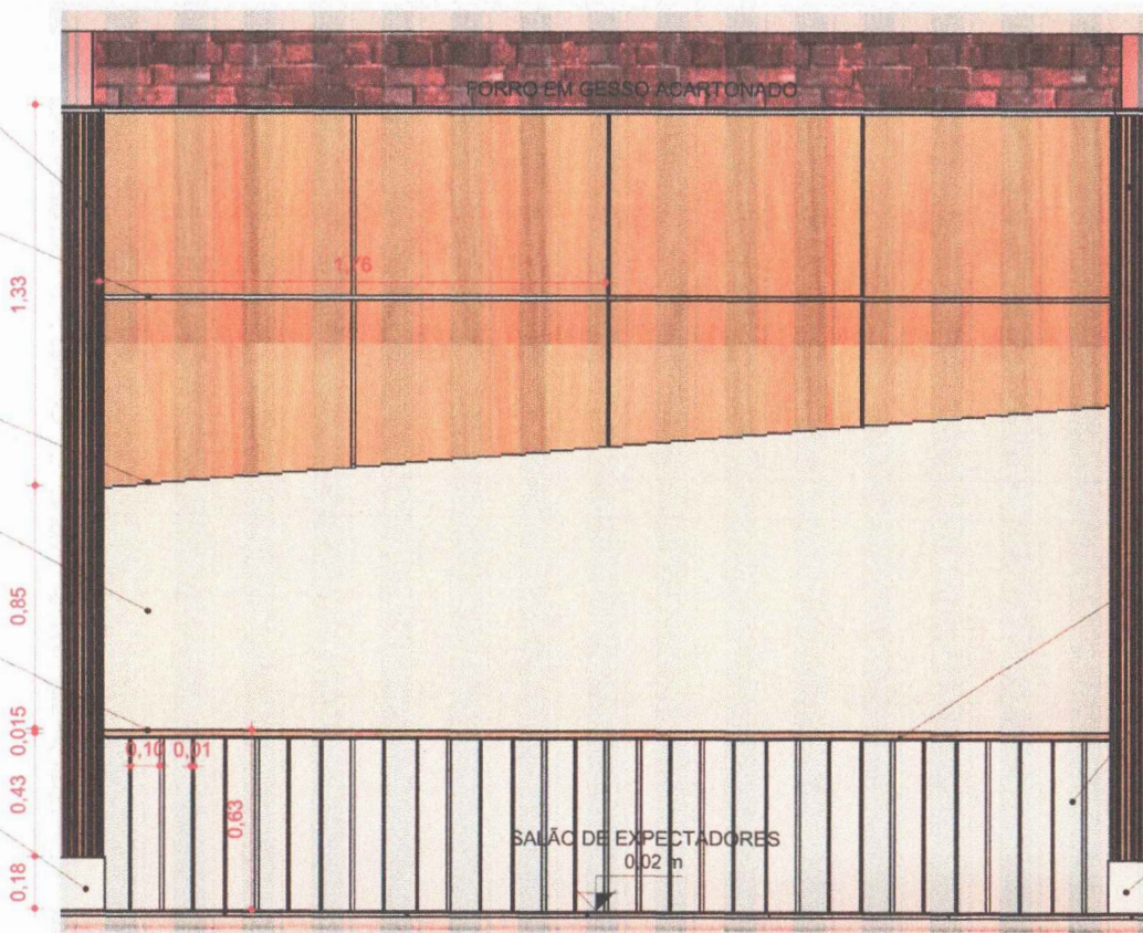
01 DETALHE - D07 1 : 20
