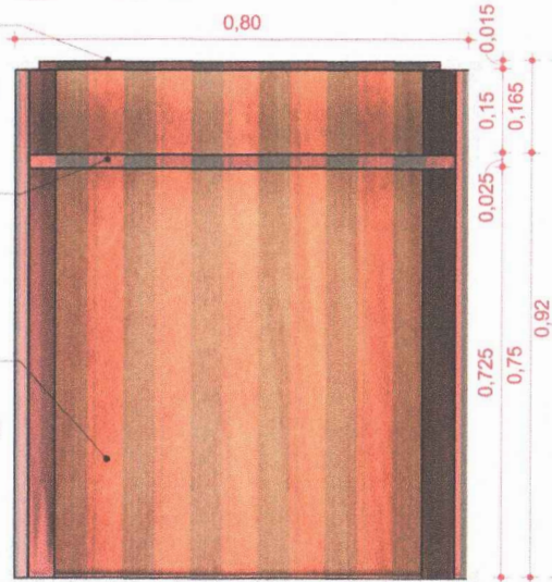
03 VISTA POSTERIOR 1 : 10
