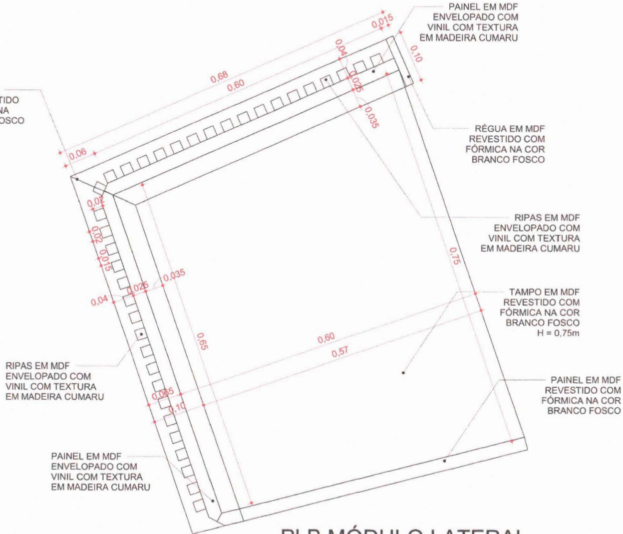
01 PLB MÓDULO LATERAL 1 : 5
