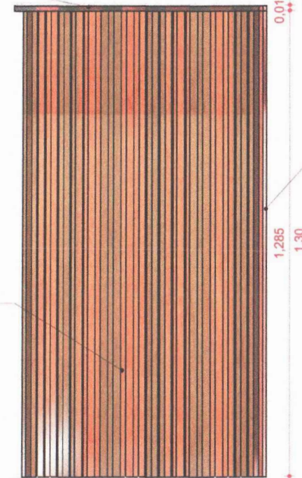
02 VISTA ESQUERDA 1 : 10
