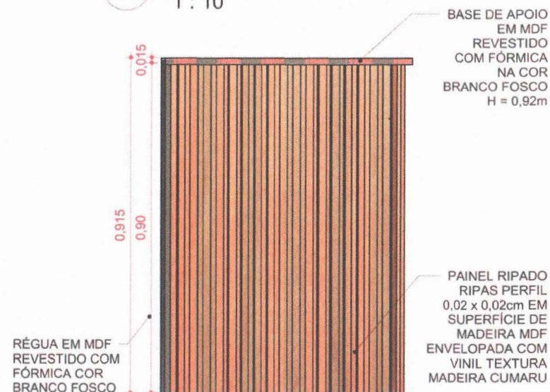
05 VISTA DIREITA 1 : 10
