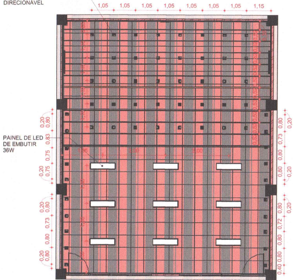
01 FORRO E LUMINÁRIAS 1:75
