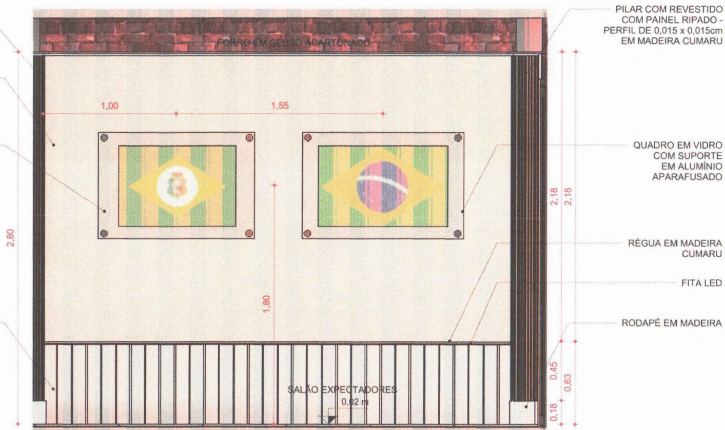
01 DETALHE - D10 1 : 20
