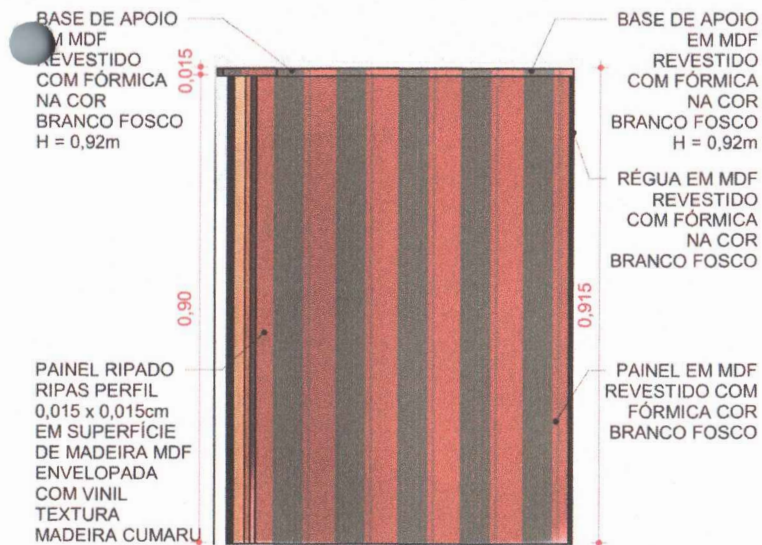
04 VISTA ESQUERDA 1 : 10
