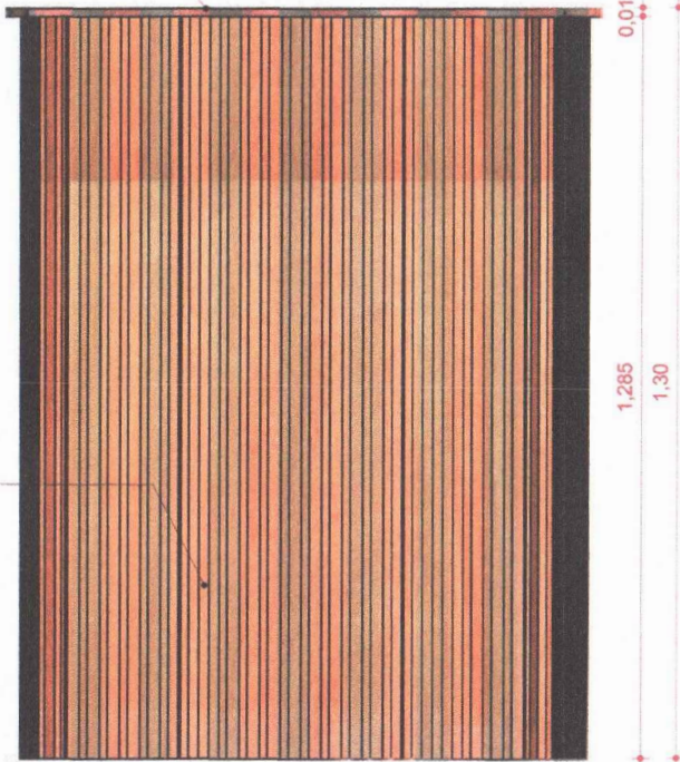
01 VISTA FRONTAL 1 : 10
