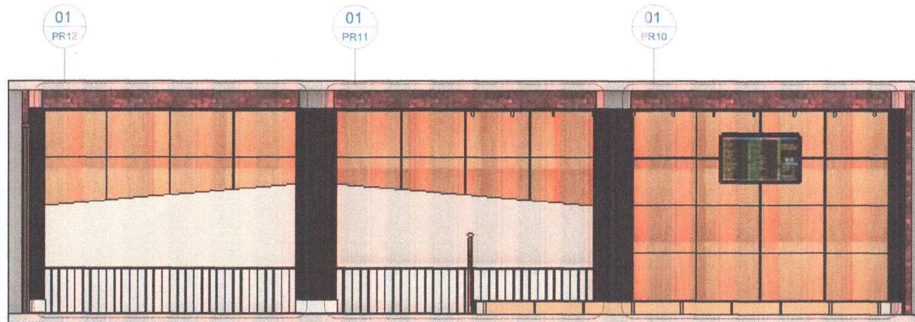
02 ELEVÇÃO 02 1 : 50
