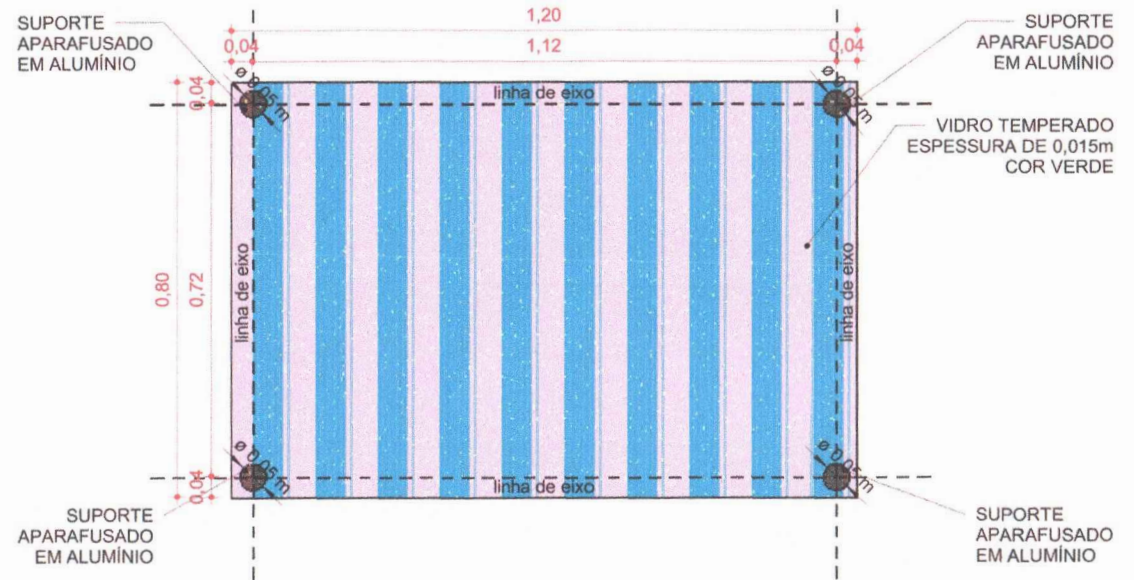
02 VISTA FRONTAL 1 : 10
