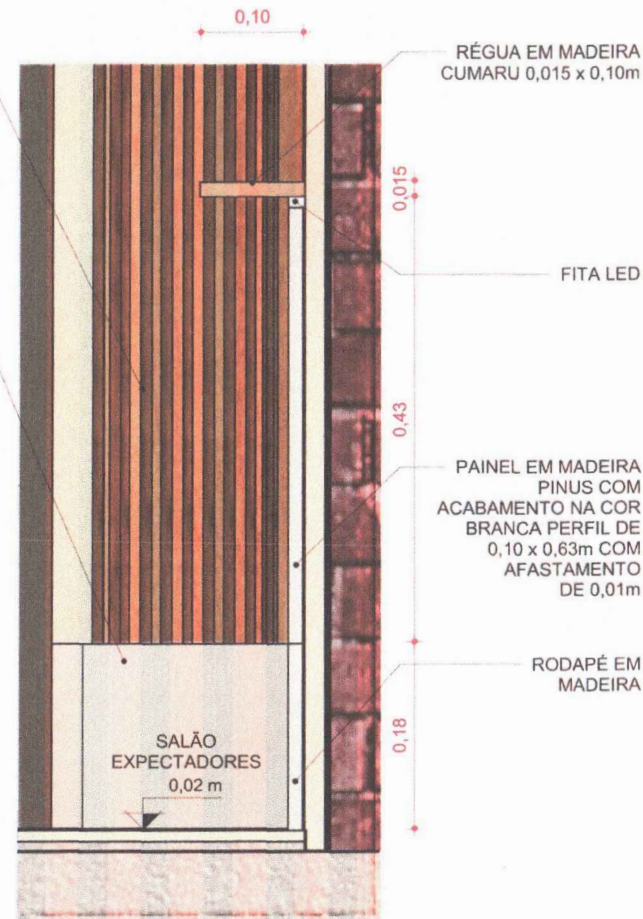
03 DETALHE - D13 1:5
