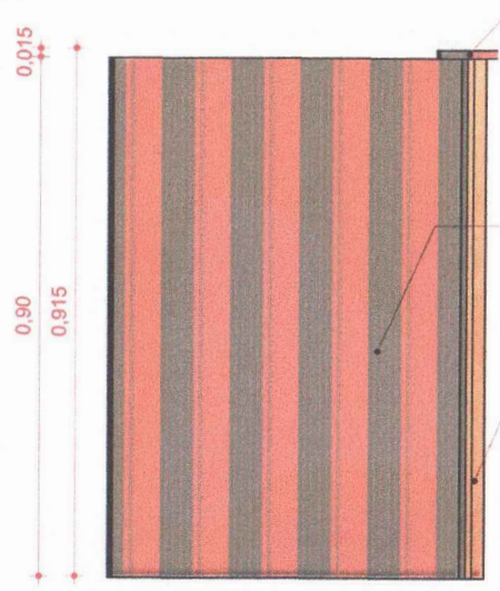
05 VISTA DIREITA 1 : 10
