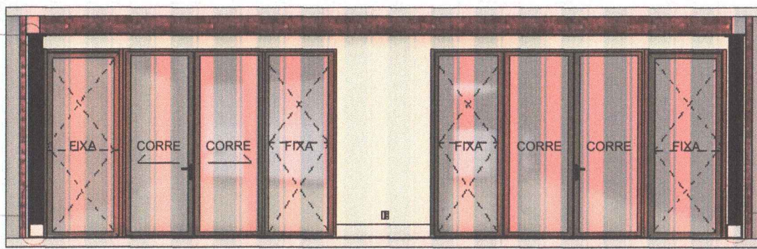
02 ELEVÇÃO 04 1 : 50
